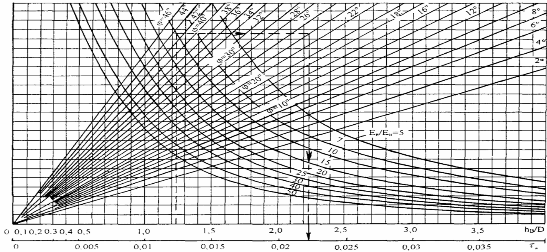
Рис. 3.3. Номограмма для определения активного напряжения сдвига от временной нагрузки в нижнем слое двухслойной системы (при h_0/D = 0 \div 4,0 )
