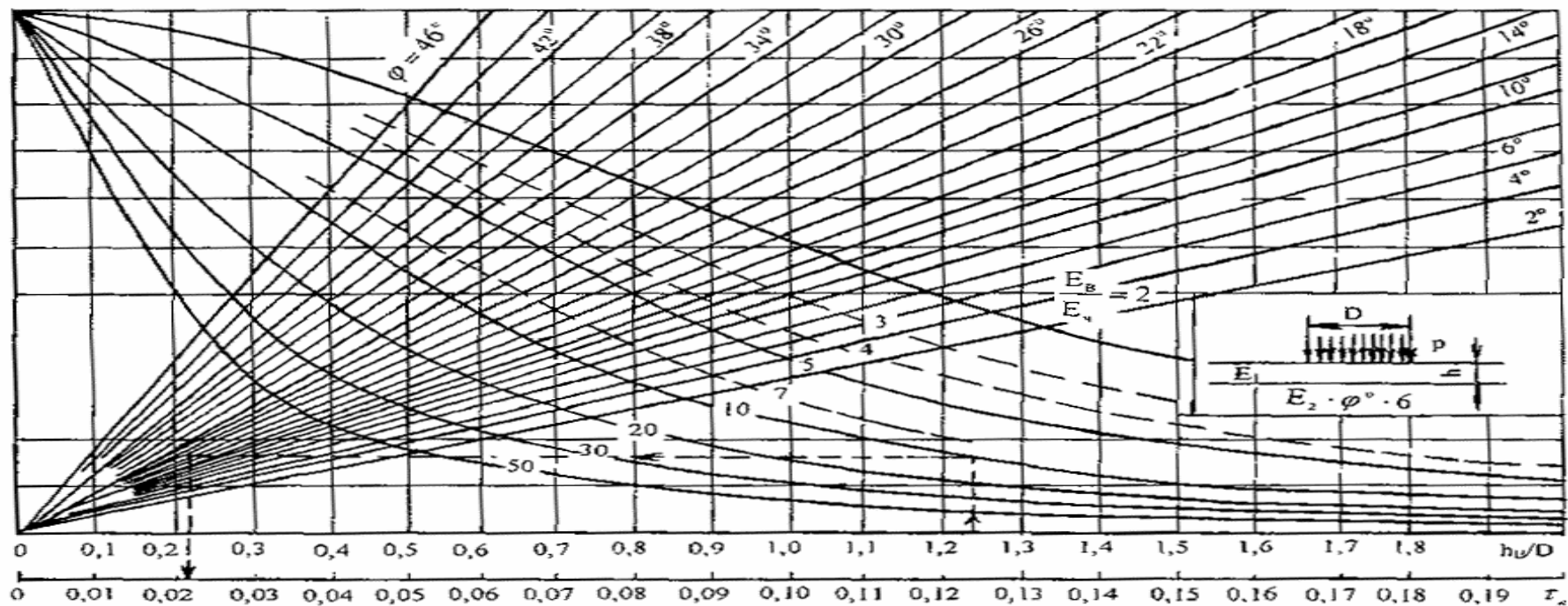
Рис. 3.2. Номограмма для определения активного напряжения сдвига от временной нагрузки в нижнем слое двухслойной системы (при h_u/D = 0 \div 2,0 )
