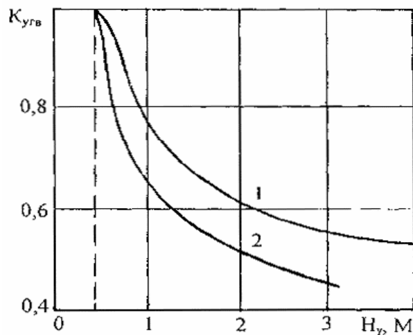
Рис. 4.1. Зависимость коэффициента K_{угв} от расстояния от низа дорожной одежды до расчетного УГВ или УПВ: 1 - супесь тяжелая и тяжелая пылеватая, суглинок; 2 - песок, супесь легкая и легкая крупная
