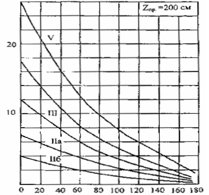
Рис. 4.3. Графики для определения осредненной величины морозного пучения I_{пуч,ср} .
