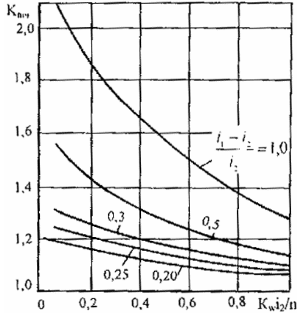
Рис. 5.3. Номограмма для определения коэффициента K_{воз} увеличения объема воды в дренирующем слое в местах изменения вогнутого профиля: i_1, i_2 - продольные уклоны выше и ниже перелома профиля; K_\phi - коэффициент фильтрации, м/сут; n - коэффициент пористости дренирующего слоя
