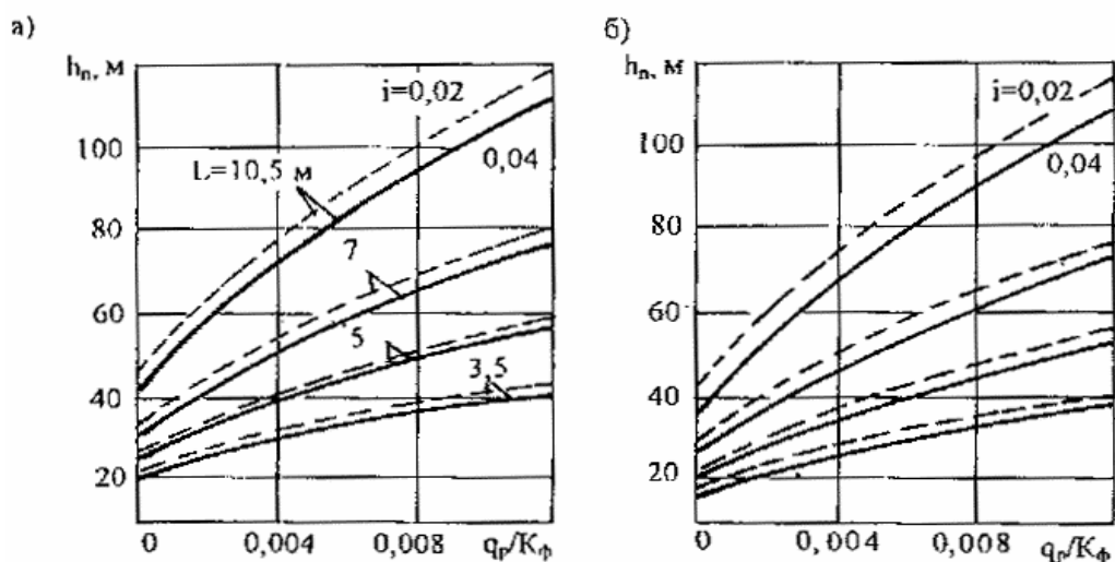
Рис. 5.4. Номограмма для расчета дренирующего слоя в конструкции с прикромочным дренажем:
