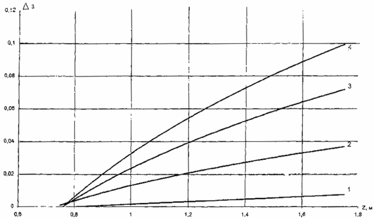
Рис. П.2.1. Графики для определения поправки на влияние суммарной толщины стабильных слоев одежды:
