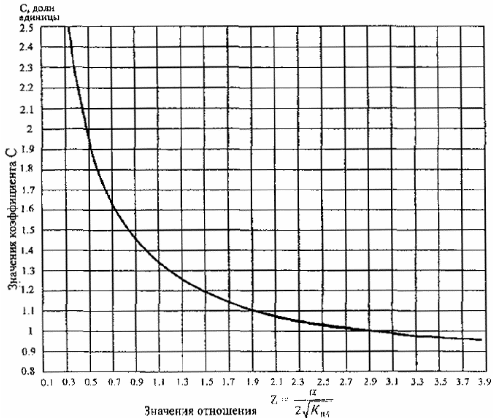
Рис. П. 7.3. График для определения коэффициента C , используемого для вычисления весенней влажности
