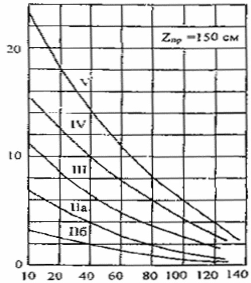
Рис. 4.3. Графики для определения осредненной величины морозного пучения I_{пуч,ср} .
