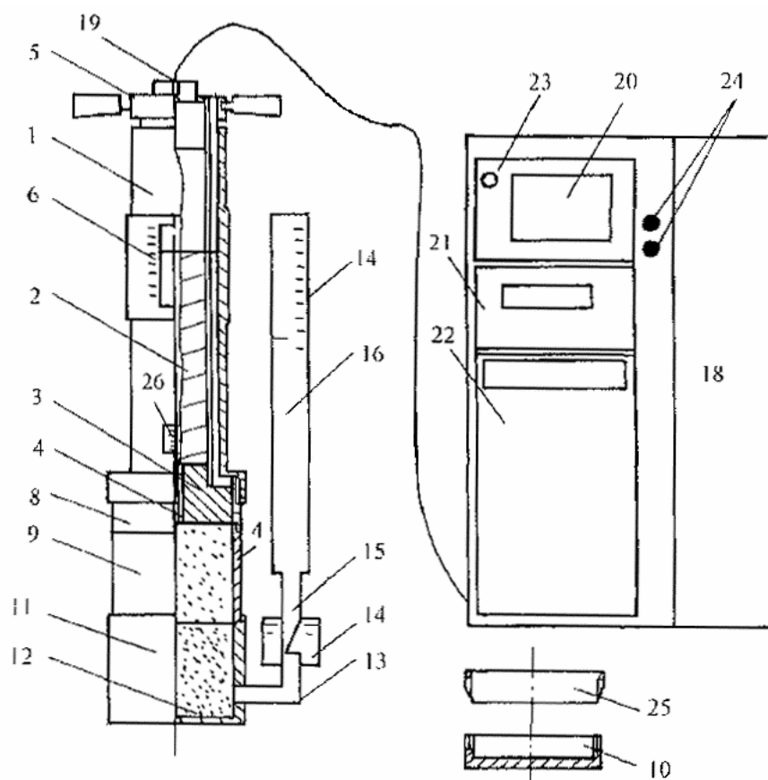
Рис. П.7.1. Схема прибора для определения коэффициента влагопроводности грунта: 1 - трубка; 2 - тарированная пружина; 3 - уплотняющий штамп; 4 - плоский электрический датчик влажности; 5 - рукоятки с винтом; 6 - измерительная шкала пружины; 7 - разъемный цилиндр-грунтонос; 8 - верхняя насадка цилиндра-грунтоноса; 9 - центральная часть цилиндра-грунтоноса; 10 - съемная днищевая крышка цилиндра-грунтоноса; 11 - форма для фильтра; 12 - крупный песок; 13 - соединительная трубка; 14 - питающая камера; 15 - подкожная трубка; 16 - питающий сосуд; 17 - водомерная шкала; 18 - регистрирующий прибор; 19 - разъем трубки; 20 - микроамперметр; 21 - таймер; 22 - микроОБМ; 23 - световой индикатор; 24 - регулировочные ручки измерительного моста; 25 - режущая кромка для отбора проб грунта ненарушенной структуры; 26 - нижняя кромка трубки
