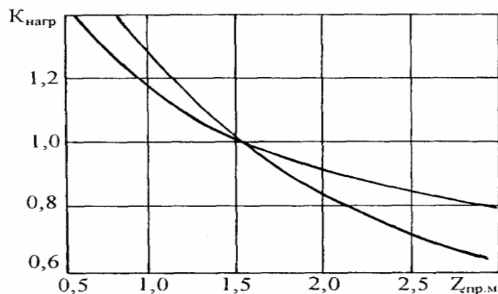
Рис. 4.2. Зависимость коэффициента K_{нагр} от глубины промерзания z_{пр} от поверхности покрытия: 1 - супесь тяжелая и пылеватая; суглинок; 2 - песок; супесь легкая, крупная
