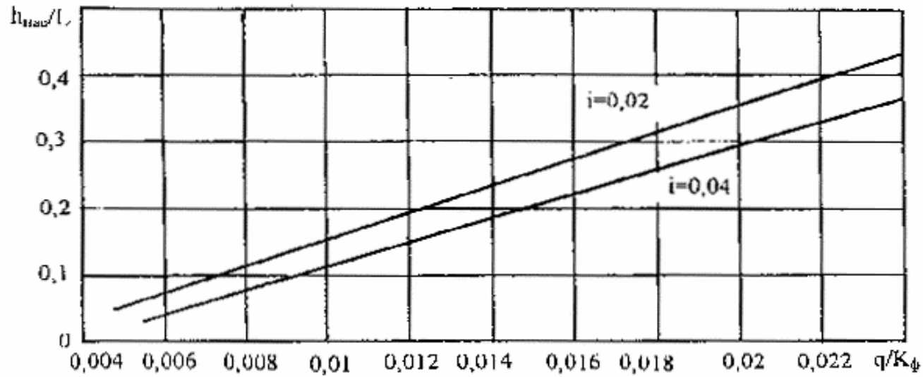
Рис. 5.1. Номограмма для расчета толщины h_{нас} дренирующего слоя из песков мелких и средней крупности, а также крупнозернистых с коэффициентом фильтрации менее 10 м/сут. При односкатном поперечном профиле q' = q_p B [м 3 /м]; при двухскатном поперечном профиле q' = 0,5q_p B [м 3 /м]; B - ширина проезжей части, м; L - длина пути фильтрации, равный B при односкатном профиле и 0,5B при двухскатном
