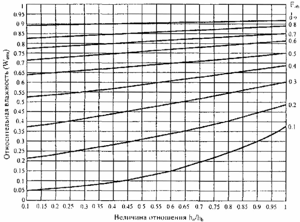
Рис. П.7.2. Номограмма для W_{отн} при значениях F_{oh} , от 0,1 до 1
