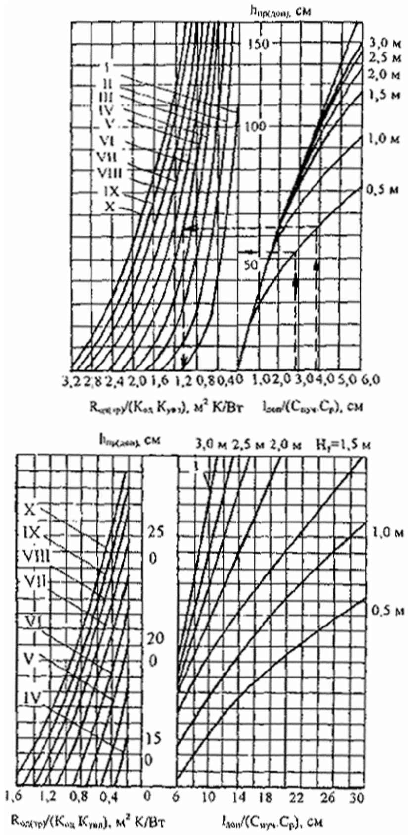
Рис 4.6. Номограмма для определения требуемого термического сопротивления дорожной одежды R_{\text{одеж(тр)}} : I-X - номера изолиний на карте (рис. 4.6); I - кривая расчета для 1-го и 2-го типов увлажнения рабочего слоя земляного полотна; H_y - глубина залегания расчетного УГВ от низа дорожной одежды, включая морозозащитные слои
