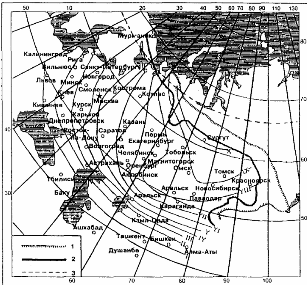
Рис. 4.5. Карта с изолиниями для определения требуемых значений термического сопротивления дорожной одежды:
