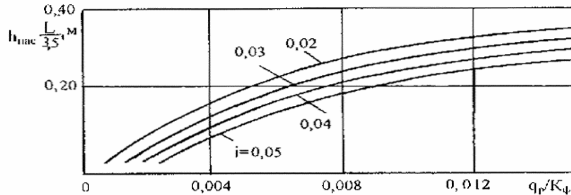
Рис. 5.2. Номограмма для расчета дренирующего слоя из крупных песков с коэффициентом фильтрации более 10 м/сут L - длина пути фильтрации в м, равная B при односкатном профиле и 0,5B при двухскатном; I - поперечный уклон низа дренирующего слоя; K_\phi - коэффициент фильтрации, м/сут
