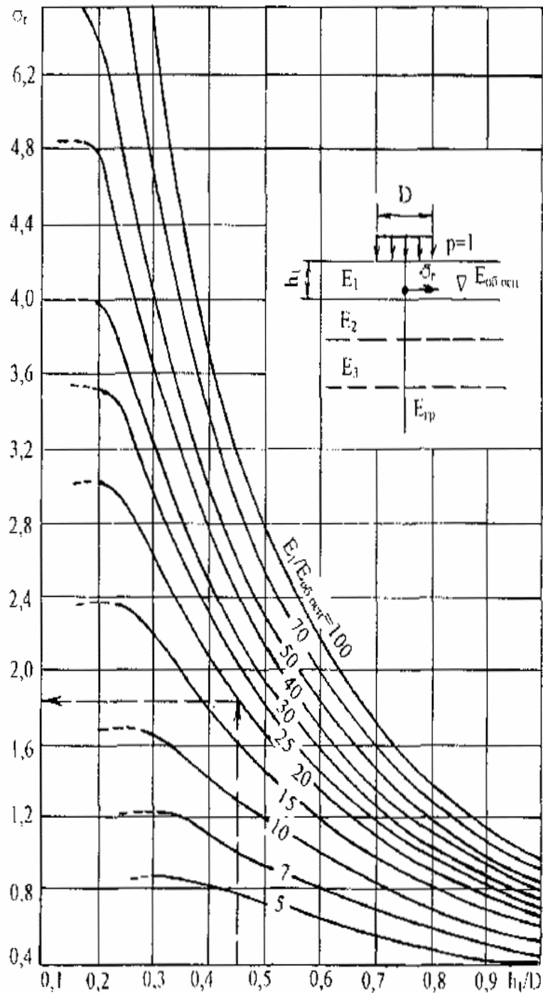
Рис. 3.4. Номограмма для определения растягивающего напряжения \sigma_r при изгибе в верхнем монолитном слое двухслойной системы
