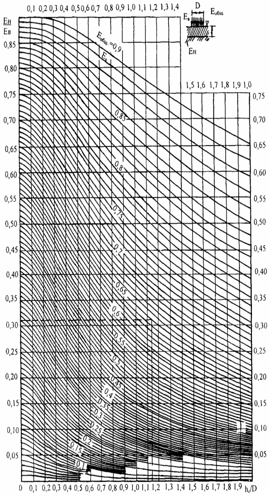
Рис. 3.1. Номограмма для определения общего модуля упругости двухслойной системы E_{общ}
